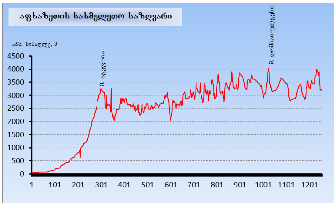
ნახ. 1.4. აფხაზეთის სახმელეთო საზღვრის ჰიფსომეტრიული პროფილი
