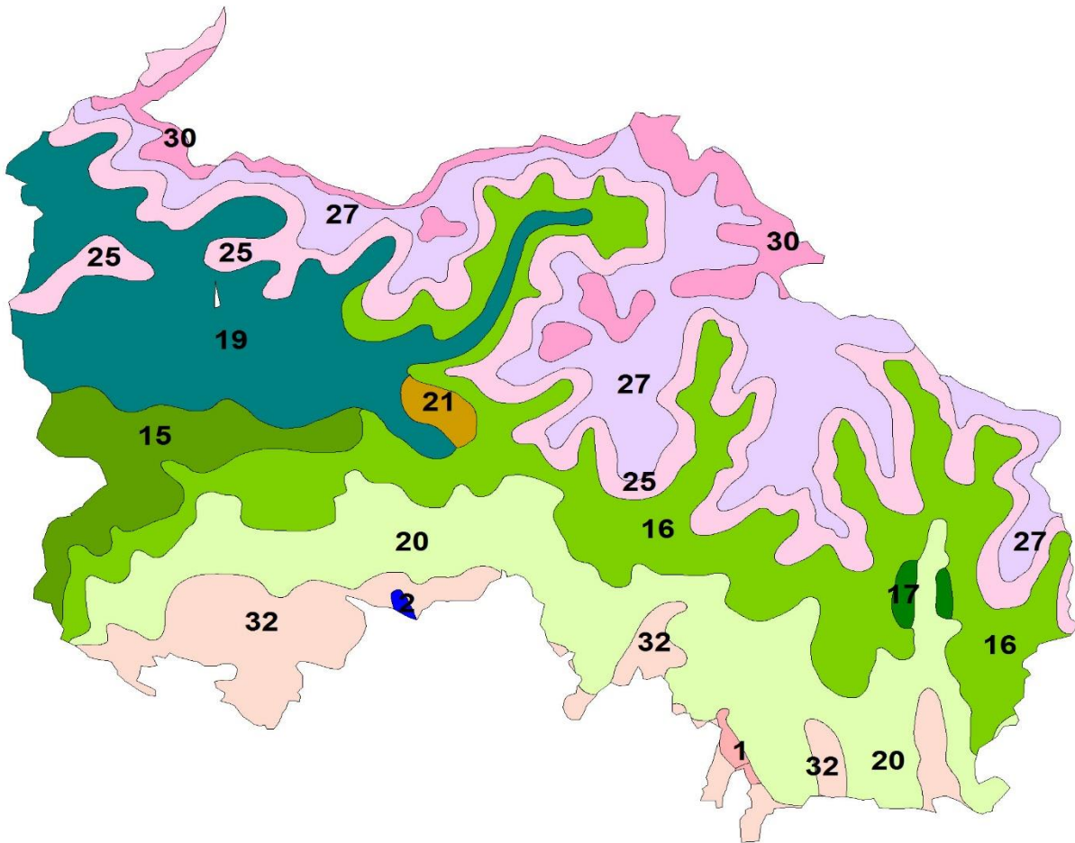
ნახ.1.4. აღდგენული მცენარეული საფარის რუკა (ნ.კეცხოველის 1958წ. მიხედვით)
