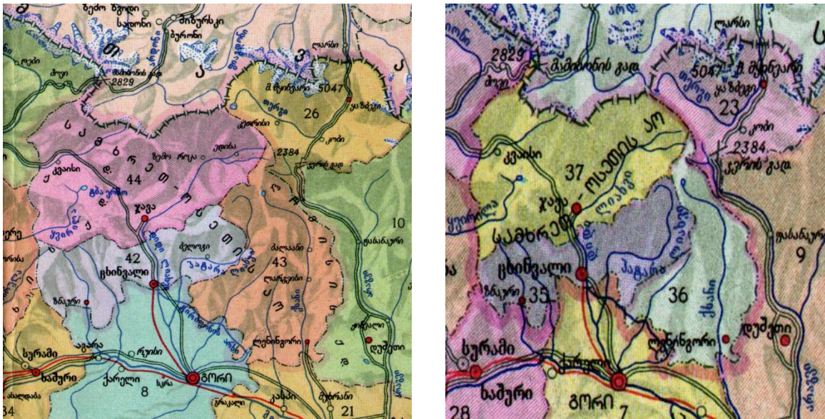
ნახ. 3.6. სამხრეთ ოსეთის ავტონომიური ოლქი 1963-1964 წლებში
