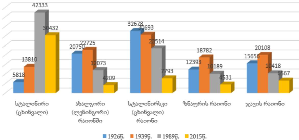
მოსახლეობის განაწილება ადმინისტრაციულ-ტერიტორიული მოწყობის მიხედვით
