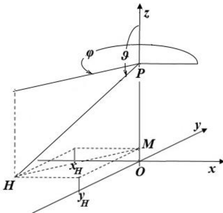
Şəkil. Hədəfin koordinatlarının təyin edilməsi sxemi
